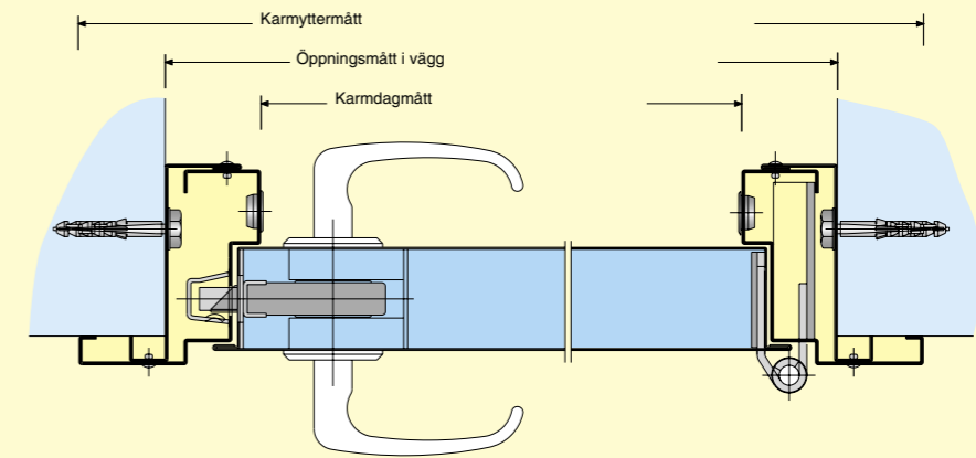
Horizontalsnitt, enkeldörr B-karm med montageprofil
