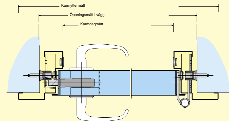
Horizontalsnitt, enkeldörr B-karm
